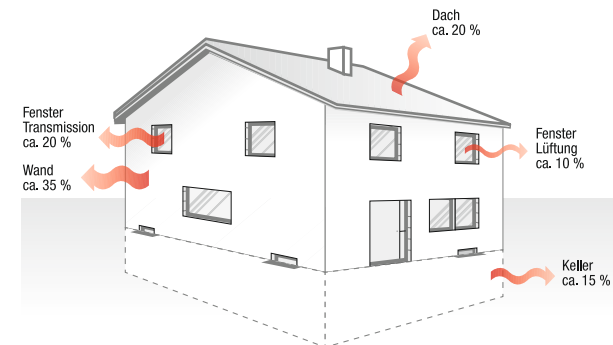
Durchschnittlicher Wärmeverlust an einem Einfamilienhaus
